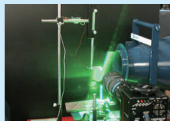
気流の可視化
